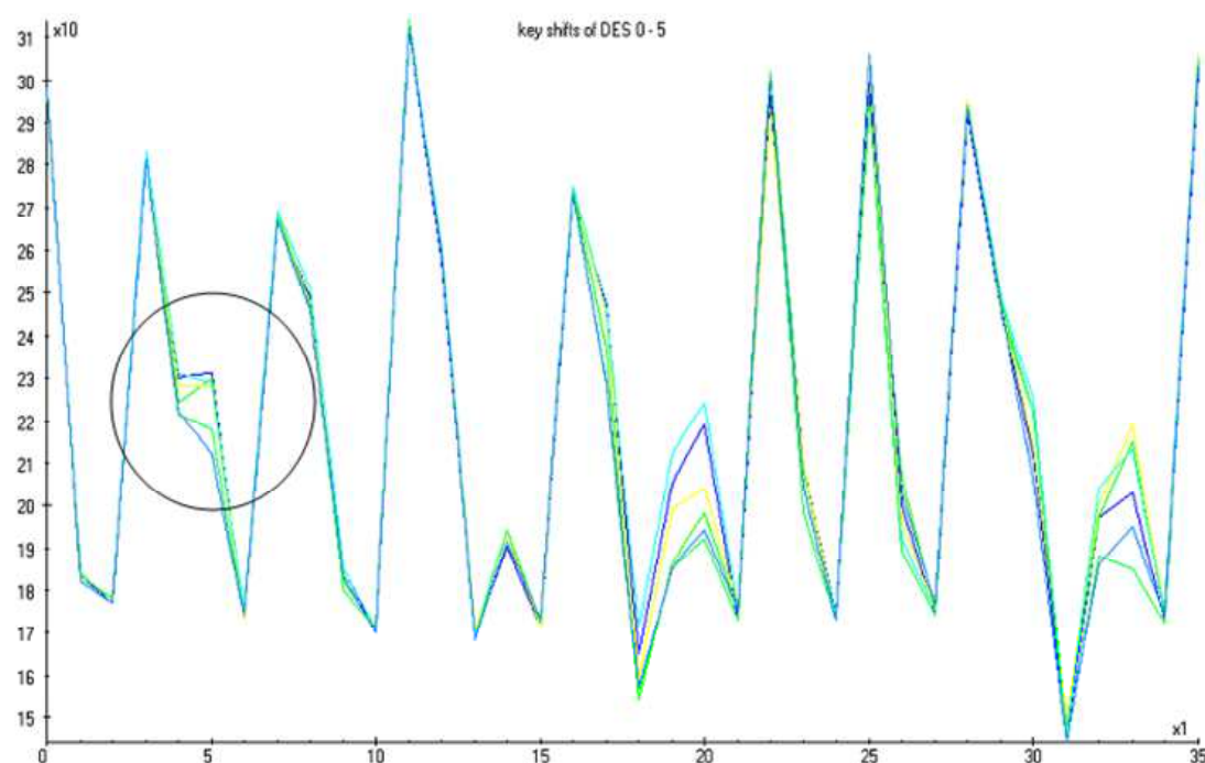
Рисунок А.8 – Различие в энергопотреблении устройства при вычислении подключа раунда алгоритма DES в зависимости от значения старшего бита ключевого регистра [115]
