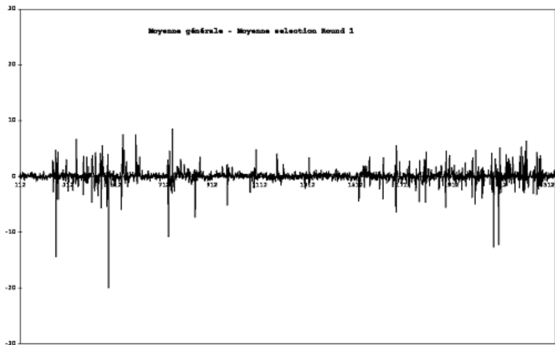
Рисунок А.9 – Разность между усреднёнными следами энергопотребления при ошибочном предположении о значении битов ключа [100]
