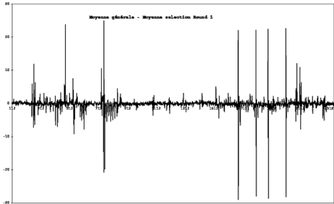
Рисунок А.10 – Разность между усреднёнными следами энергопотребления при правильном предположении о значении 6 битов ключа [100]
