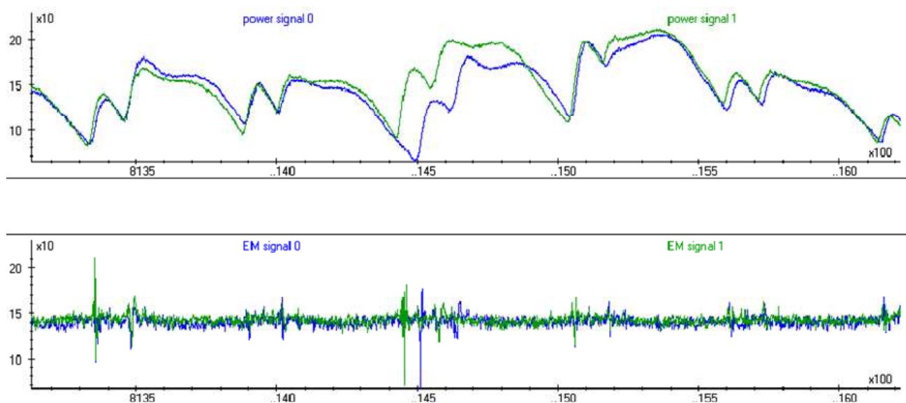
Рисунок А.11 – Сопоставление энергопотребления вычислительного устройства его электромагнитному излучению [115]
