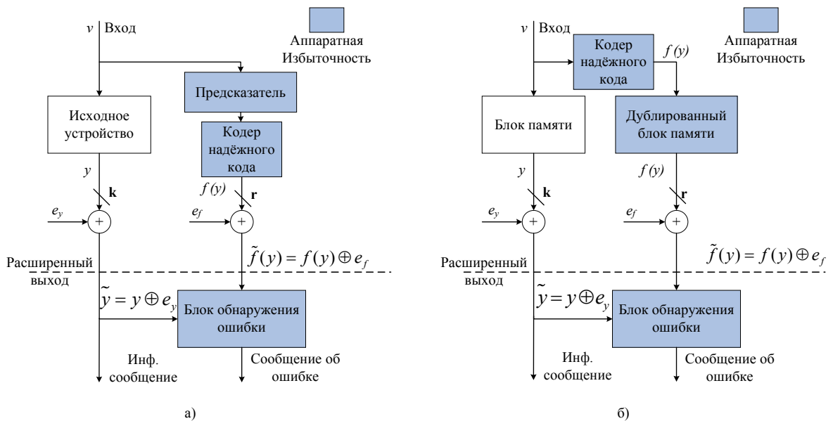
Рисунок 2.5 – Схема использования надёжных кодов для параллельного обнаружения ошибок:
