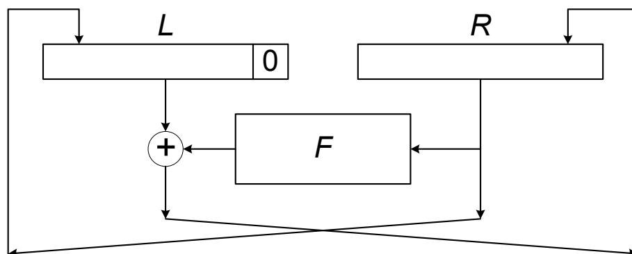
Рисунок 1.2 – Общая схема аппаратной реализации раунда DES
