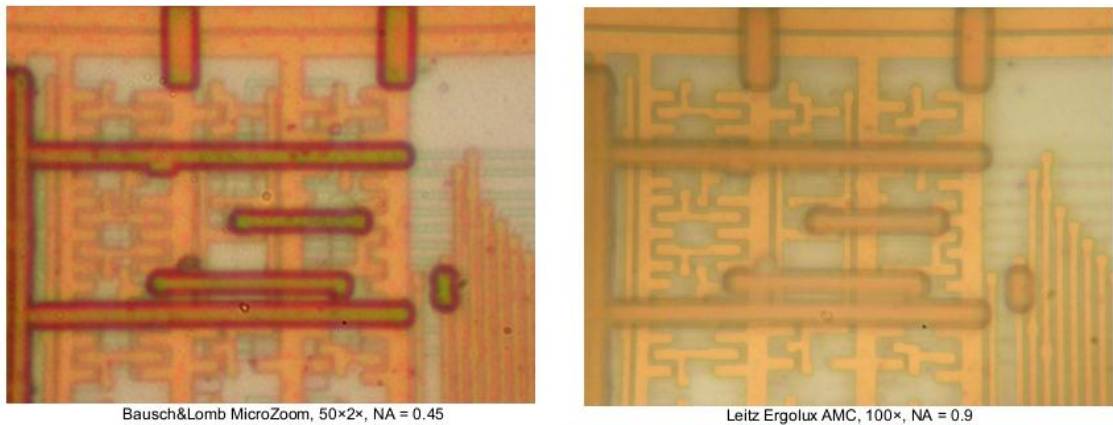
Рисунок А.4 – Изображения чипа, получаемые с помощью оптического (слева) и электронного микроскопов (справа) из [104]
