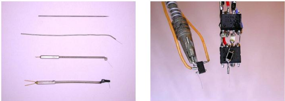
Рисунок А.5 – Щупы для подключения к чипу [104]
