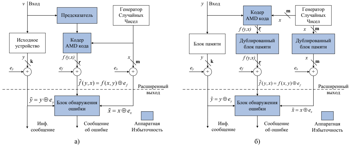
Рисунок 2.6 – Схема использования кодов, обнаруживающих алгебраические манипуляции, для параллельного обнаружения ошибок: а) для защиты линейных блоков вычислительных устройств б) для защиты блоков памяти
