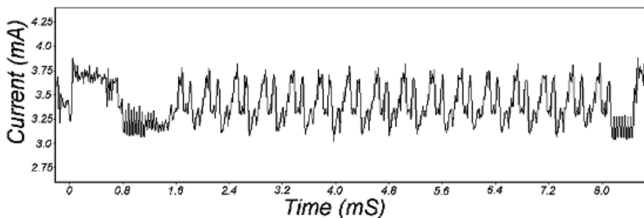
Рисунок А.7 – График энергопотребления смарт-карты, реализующей DES [113]
