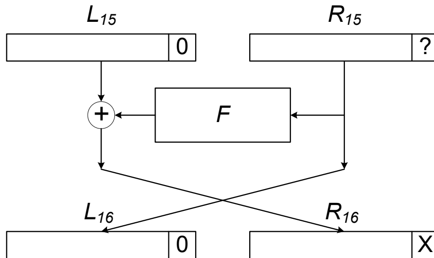
Рисунок 1.3 – Заключительный раунд DES
