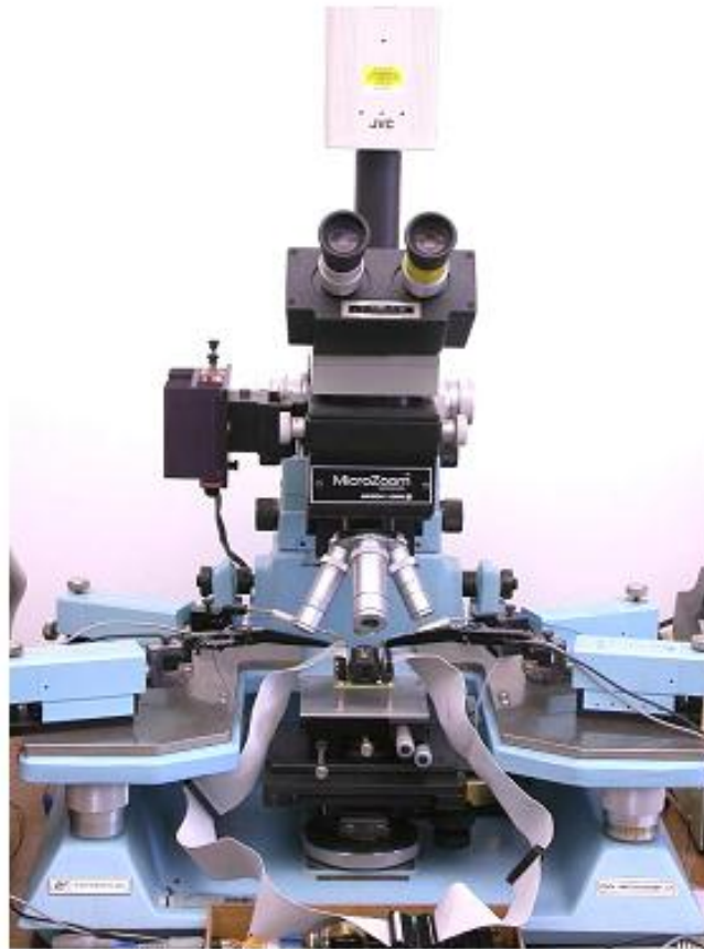
Рисунок А.6 – Пример зондирующей установки из [104]
